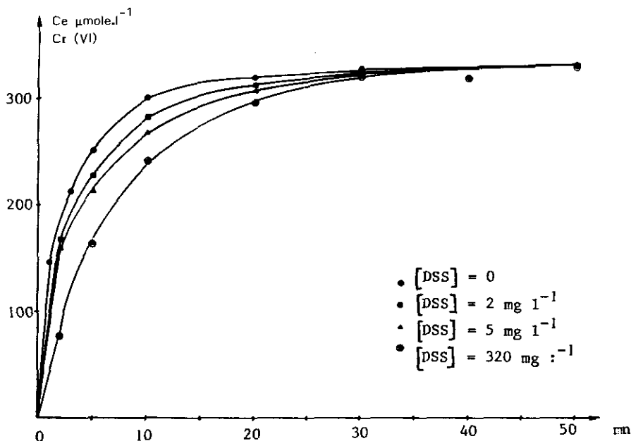
Figure 7.- Influence du DSS sur la cinétique d'échange du Cr (VI) ( 334 \text{ } \mu\text{mole.l}^{-1} ) sur les celluloses greffées AE 2 , \text{Cl}^- ( 10 \text{ g.l}^{-1} ) Ce = concentration échangée en Cr (VI).
