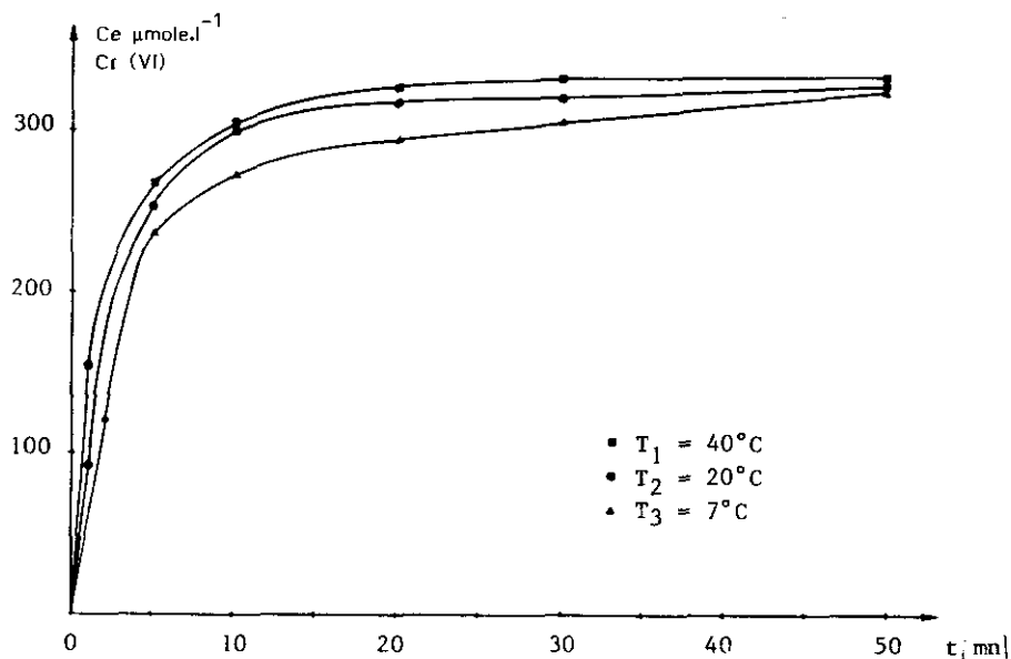
Figure 3.- Influence de la température sur la cinétique d'échange du Cr (VI) (334 μmole.l -1 ) sur les celluloses greffées AE 2 (10 g.l -1 )
