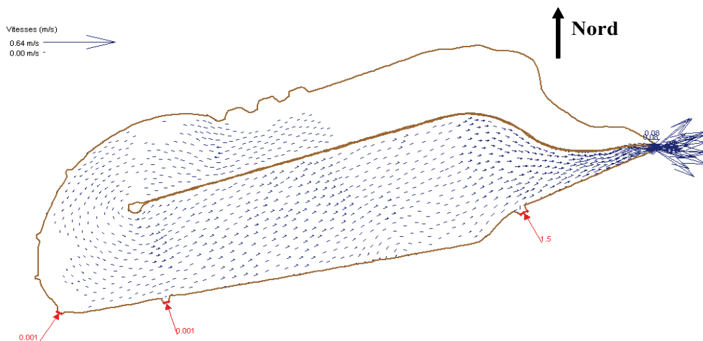
Figure 8. Champs des vitesses calculées dans le lac en marée descendante. Velocity field within the lake at ebb tide.
