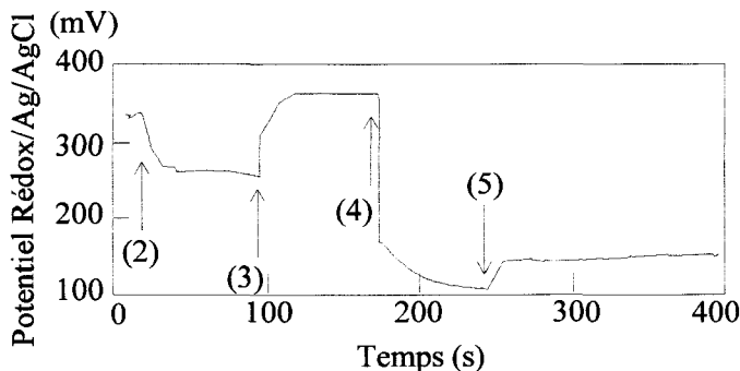
Figure 5 Potentiel redox en fonction du temps.
