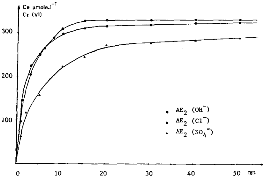
Figure 8.- Influence de l'anion des celluloses AE_2 ( Cl^- , SO_4^{2-} , OH^- ) ( 10 \text{ g.l}^{-1} ) sur la cinétique d'échange du Cr(VI) ( 334 \text{ } \mu\text{mole.l}^{-1} ) C_e = concentration échangée.
