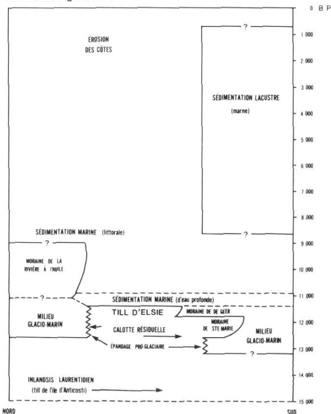
FIGURE 10. Schéma de la déglaciation. Déglaciation events.
