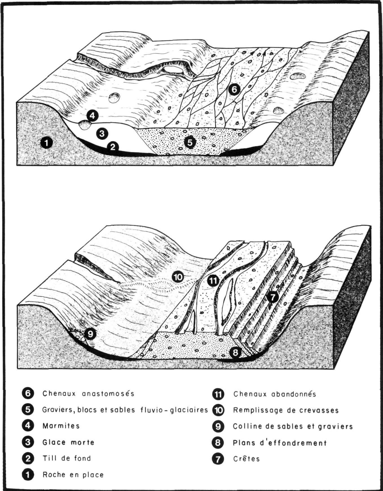
FIGURE 4. Origine des crêtes d'effondrement en bordure d'un épan-dage fluvio-glaciaire. Origin of collapsed ridges bordering glaciofluvial outwash.
