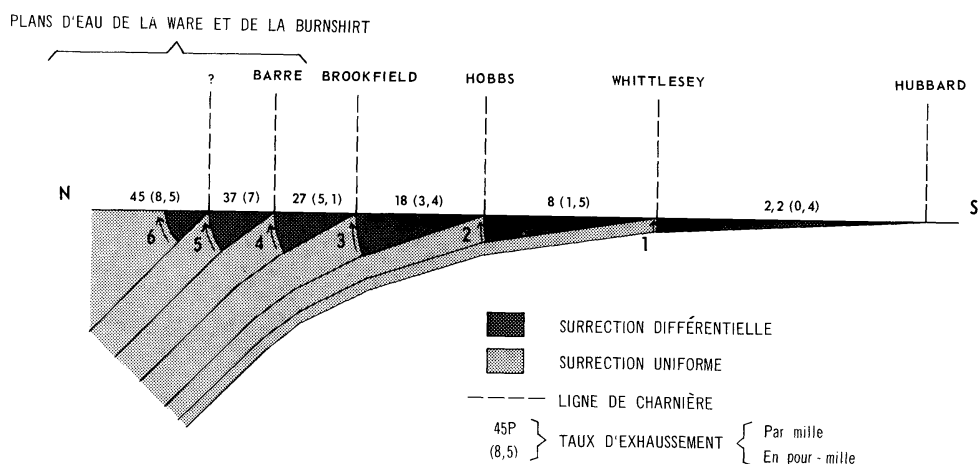
Figure 22 Diagramme schématisant comment le mécanisme de la surrection a pu jouer pour affecter la région étudiée.
