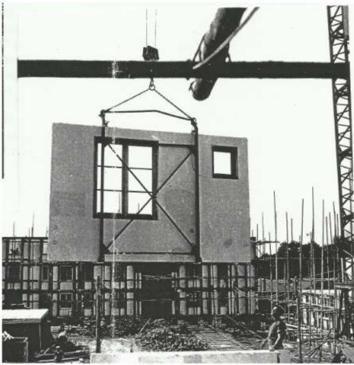
Figures 1. Pose des murs préfabriqués sur le chantier des 200 logements à Creil / Setting up the prefabricated concrete panels in the 200 houses construction site in Creil.
