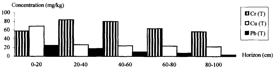
Figure 1 Évolution des teneurs métalliques totales (mg/kg) en fonction de la profondeur (cm). Metallic levels (mg/kg) evolution in terms of depth (cm).
