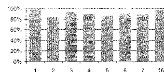
Groupes de comparaison (n = 4) Pourcentage d'accord
