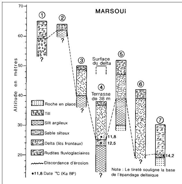
FIGURE 5. Stratigraphie des terrasses de la vallée de Marsoui. Le tireté souligne la base de l'épandage fluvi-glaciaire qui devient deltaïque à la confluence des deux vallées (rivières Marsoui et Marsoui Est). La localisation des coupes est indiquée à la figure 3.
