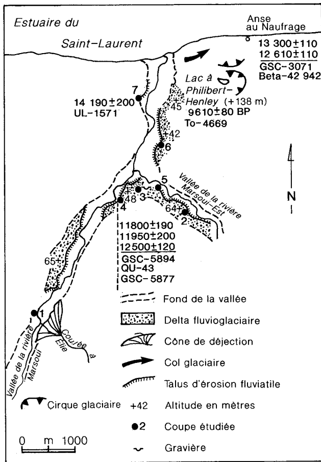
FIGURE 3. Croquis géomorphologique de la vallée de la rivière Marsouï.
