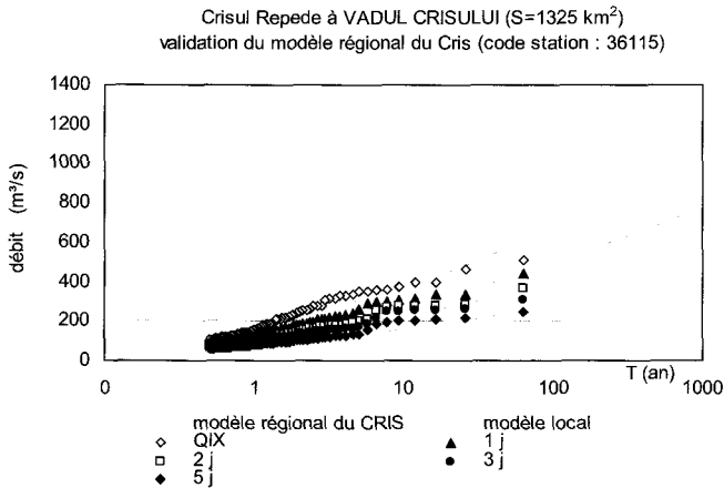
Figure 19 Exemple de validation du modèle régional du Cris (12). Validation example of Cris regional model (12).
