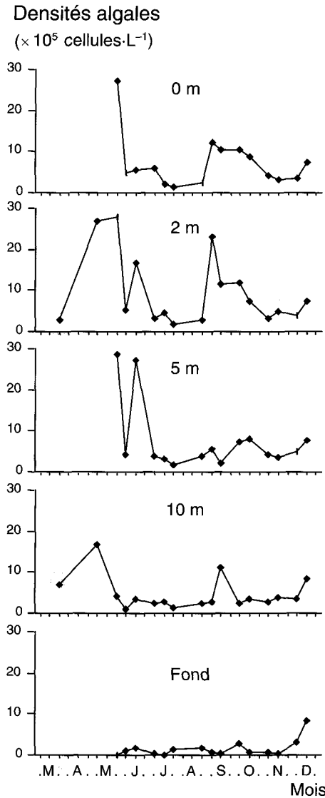
Figure 4 Variations spatiotemporelles des densités algales au niveau de la colonne d'eau. Spatial-temporal variations of algal densities at different depths of water column.
