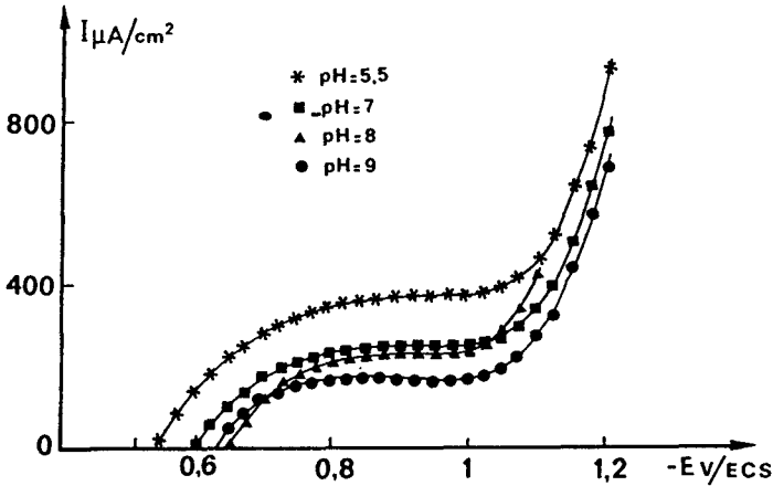
Figure 5 Courbes courant-tension cathodiques relevées en mode potentiostatique pour différentes valeurs du pH de la solution agressive, en l'absence d'inhibiteur.
