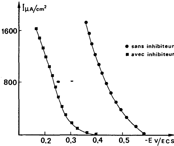
Figure 3 Courbes courant-tension anodiques relevées en mode potentiostatique en l'absence et en présence de 100 \text{ mg} \cdot \text{l}^{-1} d'inhibiteur. Anodic current-voltage curves (potentiostatic regulation) without and with inhibitor ( 100 \text{ mg} \cdot \text{l}^{-1} ).
