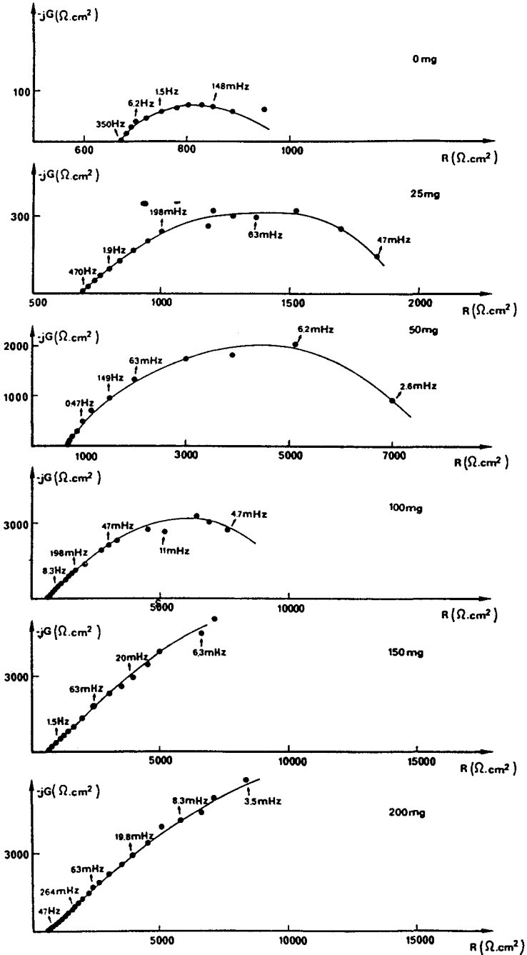
Figure 4 Diagrammes d'impédance électrochimique relevés au potentiel de corrosion pour différentes concentrations en inhibiteur (pH = 7). Electrochemical impedance diagrams corresponding to potentiostatic regulation for different inhibitor concentrations (pH = 7).
