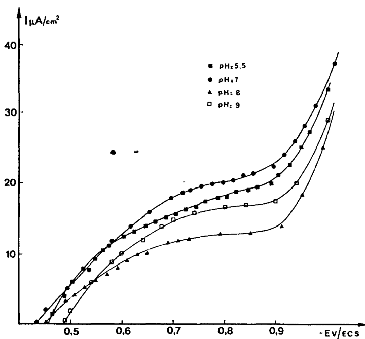
Figure 6 Idem figure 5 en présence de 100 \text{ mg} \cdot \text{l}^{-1} d'inhibiteur. Idem figure 5 with inhibitor ( 100 \text{ mg} \cdot \text{l}^{-1} ).
