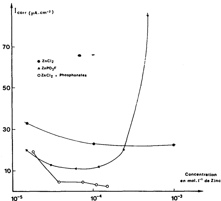
Figure 8 Variation de la vitesse de corrosion en fonction de la concentration molaire de zinc pour différents inhibiteurs.
