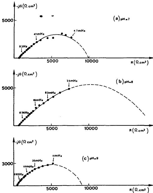
Figure 7 Diagrammes d'impédance électrochimique relevés au potentiel de corrosion pour différentes valeurs du pH de la solution.
