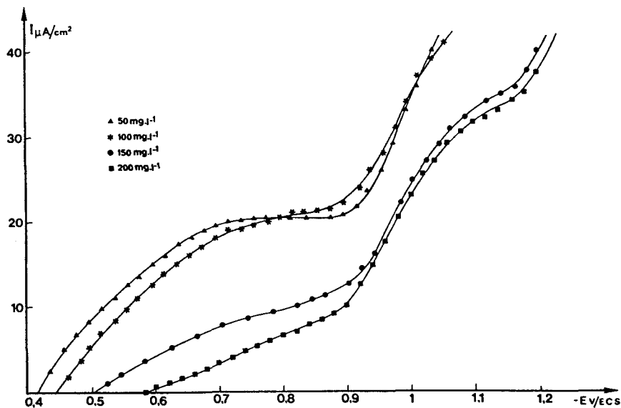
Figures 1 et 2 Courbes courant-tension cathodiques relevées en mode potentiostatique pour différentes concentrations en inhibiteur. Interface acier XC 35/NaCl 200 mg · l -1 . Cathodic current-voltage curves (potentiostatic regulation) plotted for different inhibitor concentrations.
