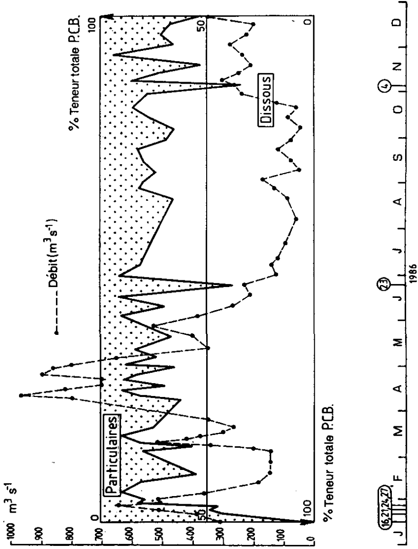
Figure 6.- Répartition de P.C.B. entre phase dissoute et phase adsorbée en pourcentage de la concentration dans l'eau brute.
