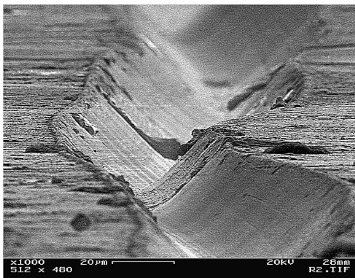
Figure 9 : Vue d'un sillon au microscope.
