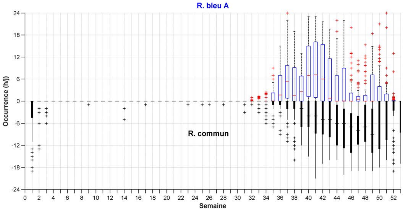
Figure 7. Diagrammes en boîtes à moustaches des statistiques hebdomadaires pluriannuelles du nombre d'heures par jour avec présence de vocalisations A du roqual bleu (haut) et de sons de 20 Hz du roqual commun (bas) de 2007 à 2017. Les boîtes indiquent les valeurs interquartiles (du 25 e au 75 e percentile); la barre centrale indique la médiane, les traits verticaux correspondent à 99 % de la distribution normale et les symboles «+» sont des données extrêmes qui vont au-delà. Notez que l'occurrence est exprimée négativement pour le roqual commun, afin de rehausser la différence avec le roqual bleu.
