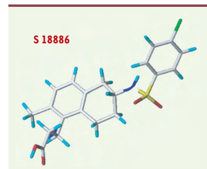
Figure 2. Structure du terutroban (S 18886).
