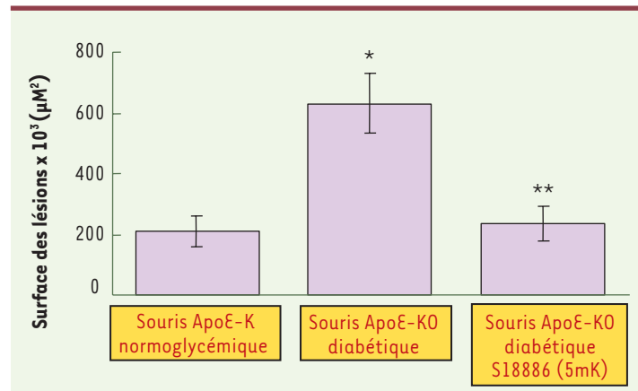
Figure 6. Le terutroban (S 18886) inhibe fortement les lésions athéromateuses dans l'aorte de souris déficientes en ApoE, rendues diabétiques. Les lésions aortiques sont plus importantes chez la souris ApoE diabétique que chez la souris ApoE. Le traitement avec le terutroban à la dose de 5 mg/kg/j (5mK) diminue fortement la formation de ces lésions. * Surface de lésions plus importante chez la souris ApoE-KO diabétique que chez la souris ApoE-KO normoglycémique ( p < 0,05 ). ** Surface de lésions moins importante chez la souris ApoE-KO diabétique traitée avec le S18886 que chez la souris ApoE-KO diabétique non traitée ( p < 0,05 ) (d'après [37]).
