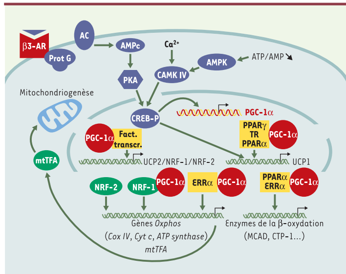
Figure 3. Implication de PGC-1 \alpha dans la biogenèse et la respiration mitochondriales, et dans l'oxydation des acides gras. Dans le tissu adipeux brun, la transcription de PGC-1 \alpha est induite après activation des récepteurs \beta_3 -adrénergiques ( \beta_3 -AR). Dans les muscles, l'expression de PGC-1 \alpha serait augmentée via les kinases dépendantes de l'AMP (AMPK) ou du calcium et de la calmoduline (CAMK IV). Une fois recruté par un facteur de transcription, PGC-1 \alpha induit l'expression de NRF-1, NRF-2 (nuclear respiratory factor 1 et 2) ou ERR \alpha (estrogen-related receptor \alpha ), d'une part, et d'une UCP (uncoupling protein), d'autre part (UCP1 dans le tissu adipeux brun, UCP2 dans les muscles). Le couple PGC-1 \alpha -ERR \alpha active seul, ou en synergie avec NRF-1 et NRF-2, selon le tissu considéré, la transcription de gènes de la chaîne respiratoire ( Oxphos ) et du facteur mtTFA (mitochondrial transcription factor) qui contrôle la transcription et la réplication de l'ADN mitochondrial. PGC-1 \alpha peut également interagir directement avec NRF-1 pour co-activer la transcription de ses gènes cibles. Enfin, PGC-1 \alpha active la transcription des gènes de l'oxydation des acides gras, en coopération avec les récepteurs PPAR \alpha ou ERR \alpha . Prot G: protéine G; AC: adénylyl cyclase; PKA: protéine kinase A; CREB: cAMP responsive element binding protein; Fact. transcr.: facteurs de transcription; PPAR: peroxisome proliferator-activated receptor; TR: thyroïd hormone receptor; Cox IV: cytochrome oxydase 4; Cyt c: cytochrome c; MCAD: medium chain acyl coenzyme A dehydrogenase; CPT-1: carnitine palmitoyl transferase 1.
