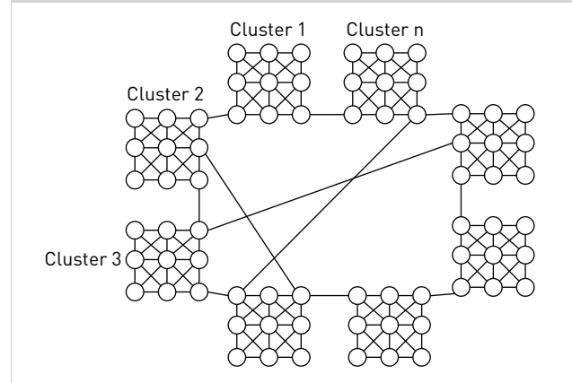
FIGURE 1 La structure du réseau en petits mondes
