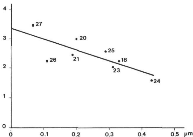
FIGURE 13. Corrélation entre le rayon moyen de la principale famille de pores ( \mu\text{m} ) et l'augmentation de longueur ( \mu\text{m}/\text{cm} ) des échantillons. Coefficient de corrélation : 0,76, significatif au seuil de 5 %.
