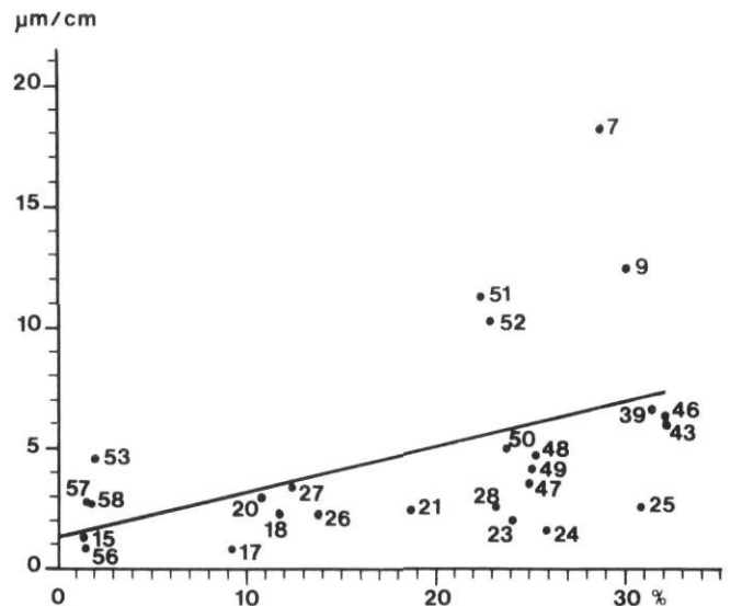
FIGURE 11. Corrélation entre la porosité (%) et l'augmentation de longueur (µm/cm) de tous les échantillons étudiés. Coefficient de corrélation : 0,49, significatif au seuil de 5 %.
