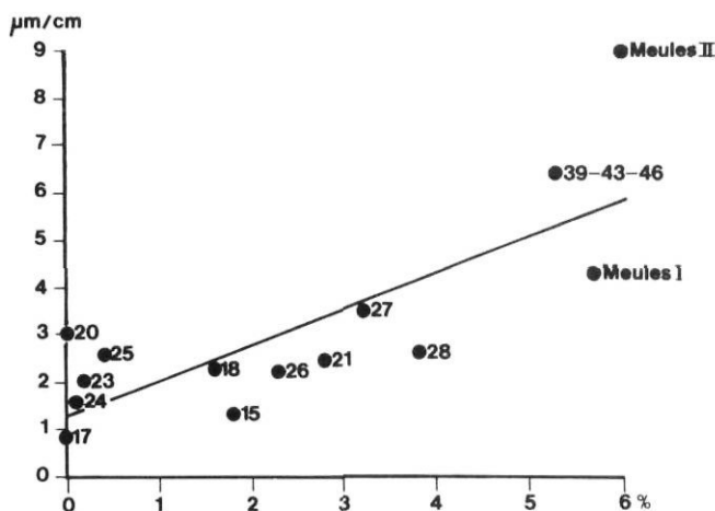
FIGURE 14. Corrélation entre la teneur en argile (%) et l'augmentation de longueur (μm/cm) des échantillons. Coefficient de corrélation : 0,79, significatif au seuil de 0,1%.
