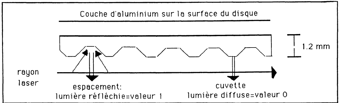
Fig.1 : CD-ROM : conversion des signaux lumineux en code binaire
