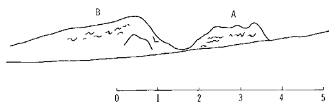
Figure 4 Coupe verticale de l'estran entre les embouchures de la rivière Géophysique et du ruisseau du Nord.
