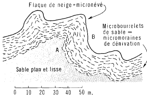
Figure 6 Micromoraines de dénivation, résultat de la fonte d'une plaque de neige mêlée de sable (B), le tout vu de dessus.
