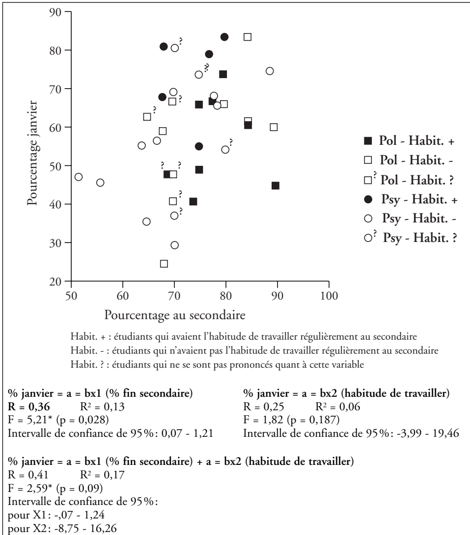
Figure 2 – Scattergramme réussite janvier – Antécédents scolaires
