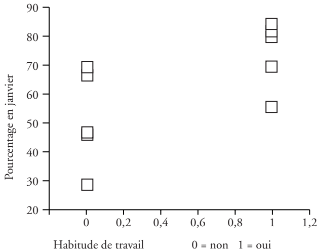
Figure 5 – Scattergramme PSY: Réussite janvier – Habitude de travailler au secondaire
