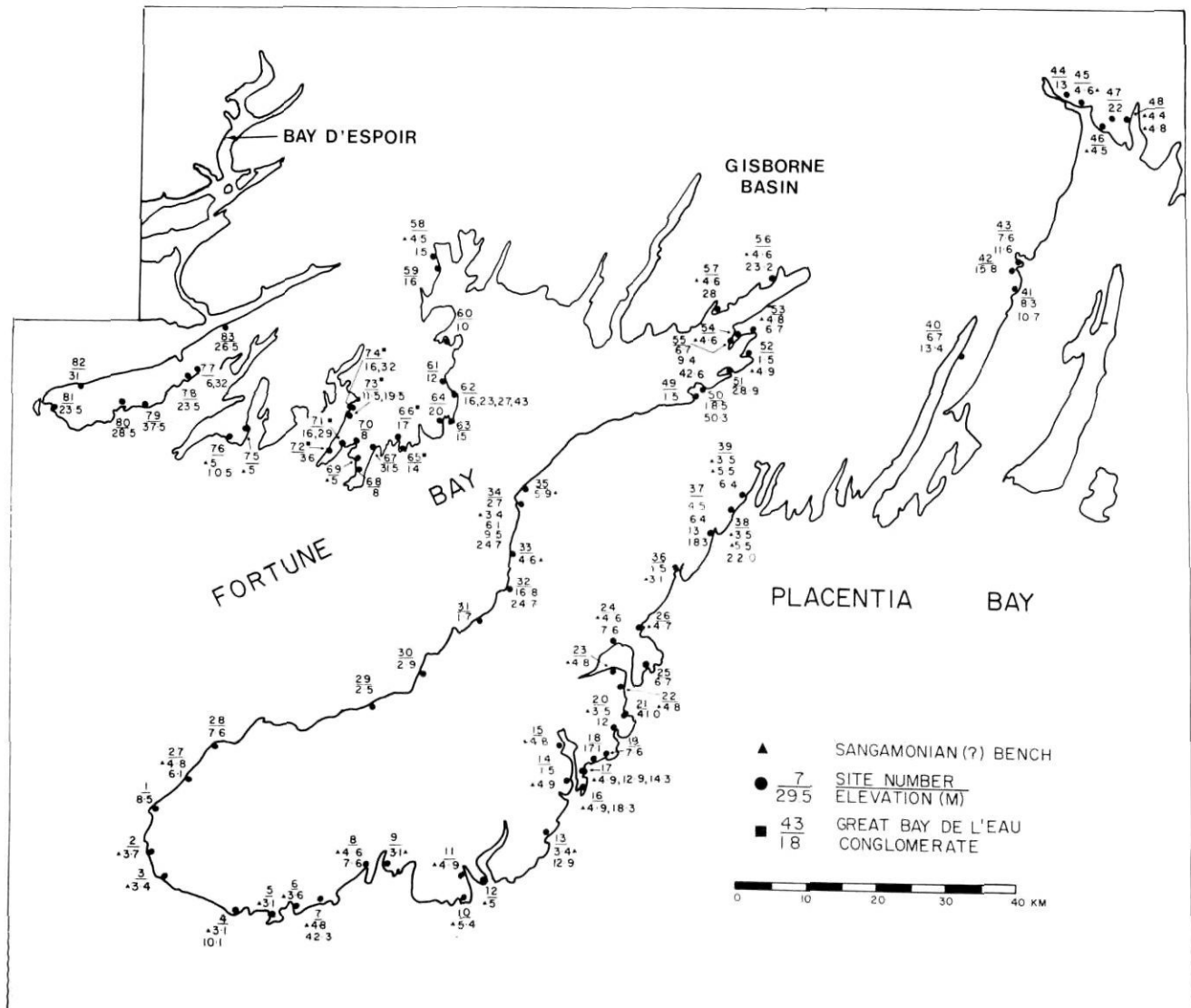
Altitudes des plates-formes marines soulevées dans la région de Burin-Hermitage au sud de Terre-Neuve. Le point de référence est le niveau le plus élevé des eaux au moment des plus fortes marées.
