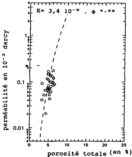
Figure 5 Relation entre la porosité et la perméabilité (mesures sur carottes). Relation between porosity and permeability (cores measurements).
