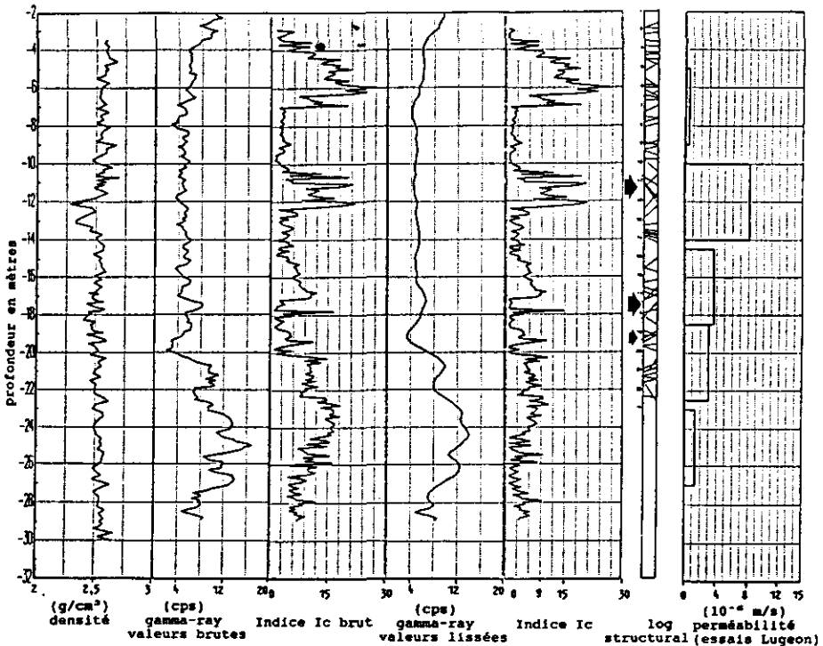
Figure 7 Profils diagraphiques du forage de Samson.
