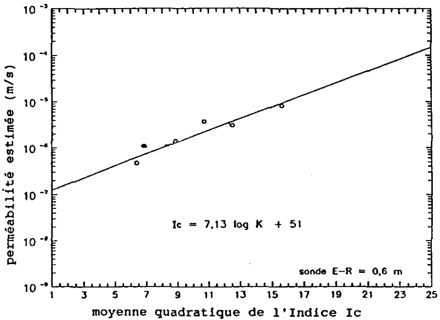
Figure 9 Relation entre la perméabilité Lugeon et la moyenne quadratique de l'indice Ic corrigé : Ic - C(Ic) . Relation between the Lugeon permeability and the quadratic average of the corrected index Ic : Ic - C(Ic) .
