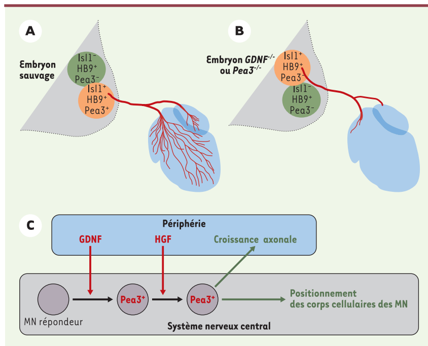
Figure 3. Intervention du GDNF et de l'HGF dans la différenciation des motoneurons (MN). Le GDNF puis le HGF, synthétisés à la périphérie, contrôlent la différenciation d'une sous population de MN en contrôlant l'expression de Pea3 . Schémas montrant le positionnement des corps cellulaires des MN ainsi que leur croissance axonale à 12,5 du développement embryonnaire dans un embryon sauvage (A) et dans un embryon mutant pour GDNF ou Pea3 (B). L'absence du signal GDNF ou Pea3 entraîne le mauvais positionnement des MN qui auraient exprimé PEA3 ainsi qu'une arborisation axonale déficiente. Pour plus de clarté, seuls les MN impliqués ont été schématisés. (C) Schéma résumant le rôle de GDNF et de HGF dans la différenciation des groupes de MN via l'expression de PEA3 [17, 20, 21].
