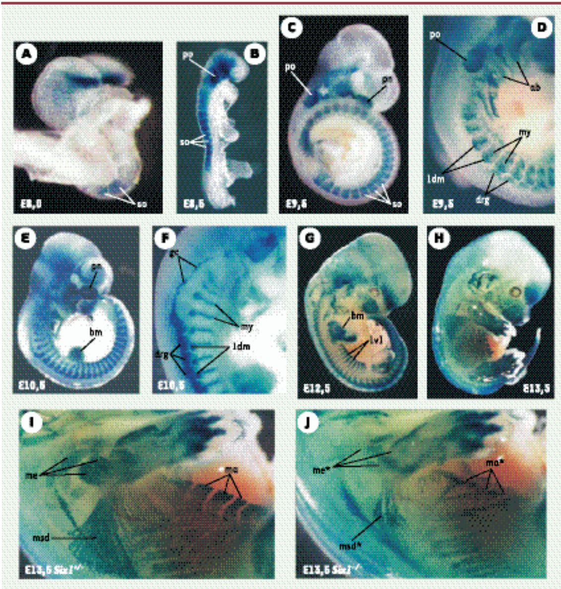
Figure 2. Profil d'expression du gène Six1 au cours du développement et phénotype musculaire des embryons Six1 -/- à E13,5 dpc.
