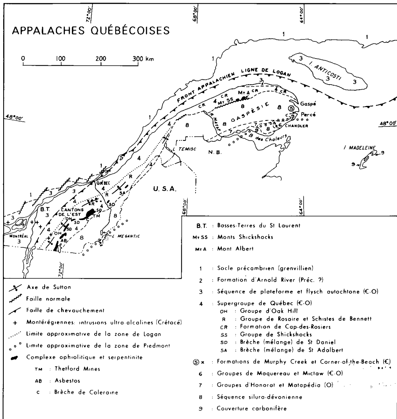
Figure 1 Carte tectonique des Appalaches du Québec.
