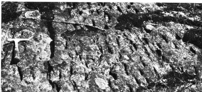
Photo 4 Alvéoles de corrosion dans anorthosite en milieu subaérien, à l'est de Saint-Ambroise ; les cavités qui sont allongées et alignées parallèlement traduisent des influences lithologiques et structurales mineures.
