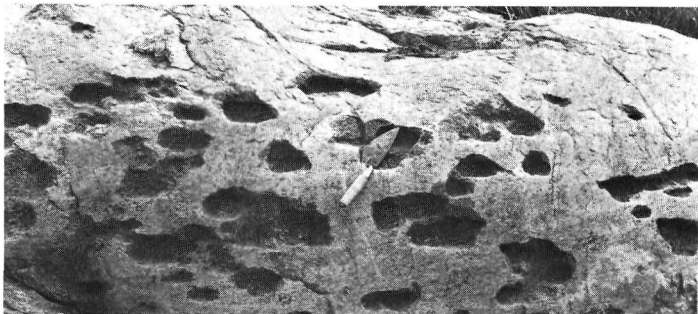
Photo 2 Alvéoles de corrosion dans anorthosite près de Saint-Coeur-de-Marie, rivage sud-est du lac Saint-Jean. Les cavités affectant une surface polie par les glaciers quaternaires sont évidemment postérieures au Pleistocène.
