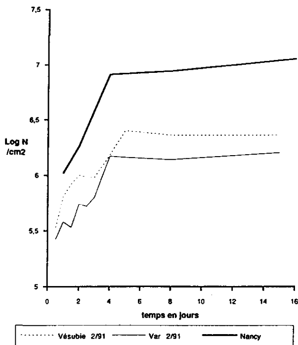
Figure 8 Colonisation des pastilles de matériel immergées dans les réservoirs. Colonization of immersed coupons of materials in the reservoirs.
