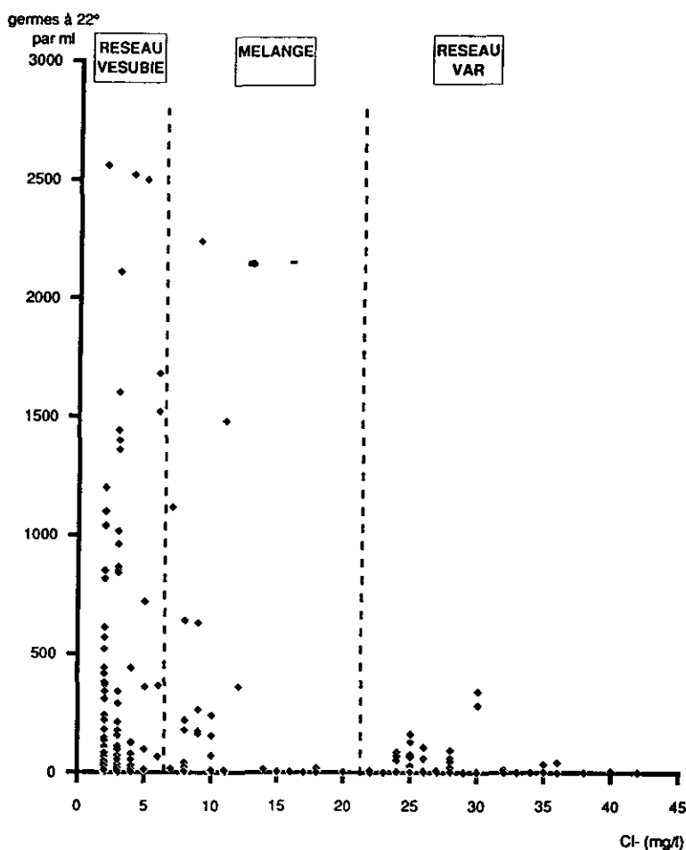
Figure 7 Germes revivifiables à 22 °C en fonction de la concentration en chlorures.
