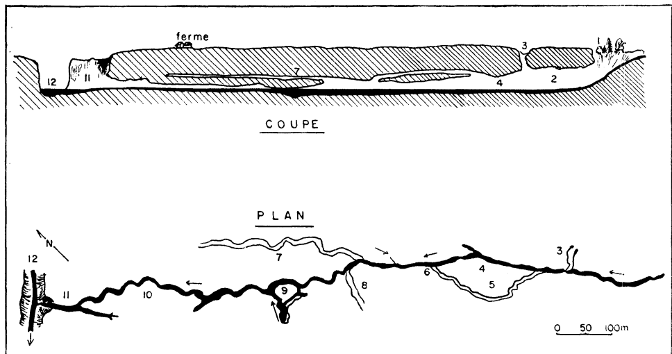
FIGURE VII GROTTE DE SAINT-CASIMIR
