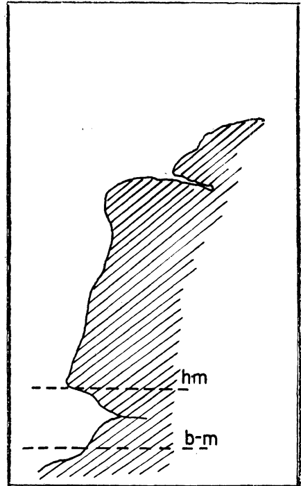
FIGURE XII PROFIL D'UNE CÔTE CALCAIRE (ÎLE SAINT-CHARLES, MINGAN)
