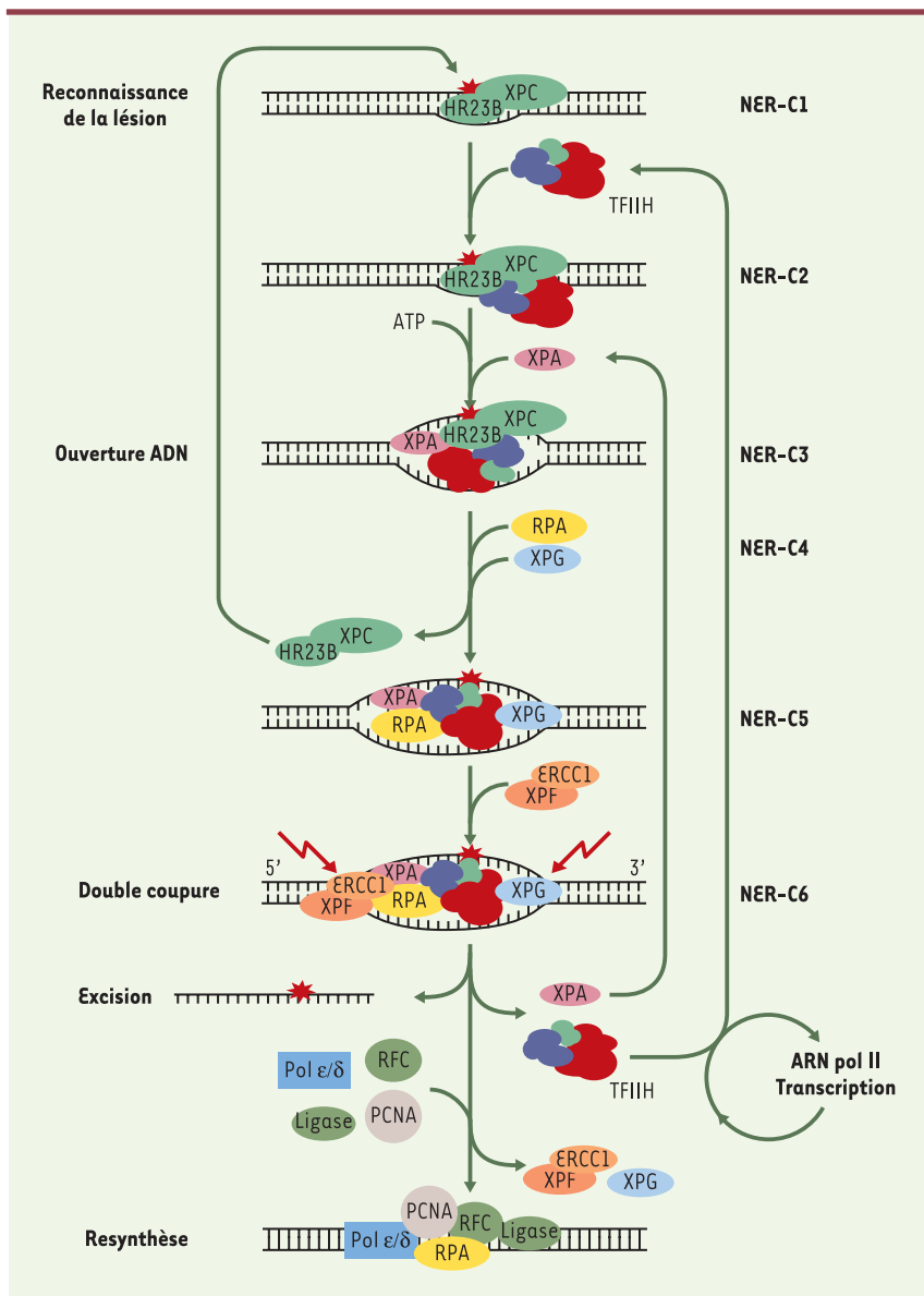
Figure 1. XPC, complexé à la protéine HR23B, interagit avec la structure formée par l'ADN endommagé (complexe NER-C1). L'entrée de TFIIH forme le complexe NER-C2. En présence d'ATP, les hélicases XPD et XPB contenues dans TFIIH déroulent la molécule d'ADN, permettant les associations séquentielles de XPA, RPA et XPG et conduisant à la formation du complexe NER-C5. L'entrée de XPG catalyse le départ et le recyclage de XPC-HR23B. Avec l'entrée de l'endonucléase XPF-ERCC1 est formé le complexe d'incision NER-C6 qui catalyse l'excision de l'oligonucléotide portant la lésion, le relargage de XPA et TFIIH. TFIIH est ainsi rendu disponible pour la formation de nouveaux complexes d'incision. En l'absence de dommage dans l'ADN, TFIIH peut aussi être re-associé avec l'ARN polymérase II. RPA, XPG et XPF-ERCC1 restent associés à l'ADN simple brin restant jusqu'à l'arrivée des facteurs de re-synthèse de l'ADN avec lesquels RPA reste associé (d'après [15]).
