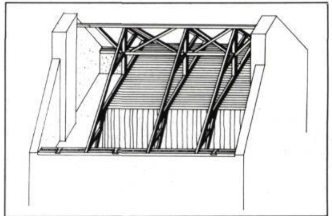
2. Exemple d'une charpente ancienne datant du Régime français. On y remarque la plupart des composantes de trois fermes contreventées par des «croix de Saint-André». (dessin: C. Diacon)
